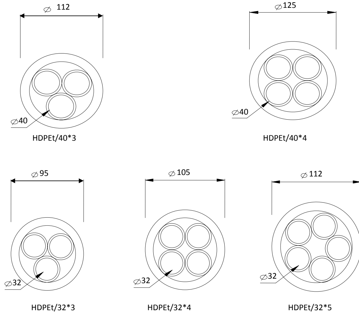
Hình 6 - Quy cách hình dáng ống nhựa HDPEt
