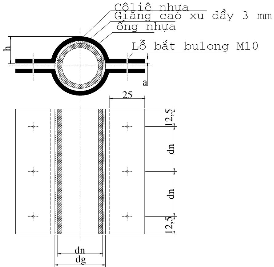
Hình 8: Bộ nối ống nhựa HDPEp kiểu coliê
