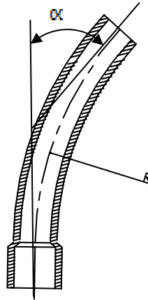
Hình 3 - Ống cong
