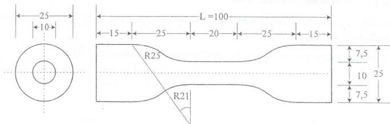
Hình A.1: Mẫu thử dạng chảy
