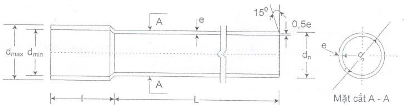
Hình 1 - Quy cách hình dáng ống nhựa PVC-U
