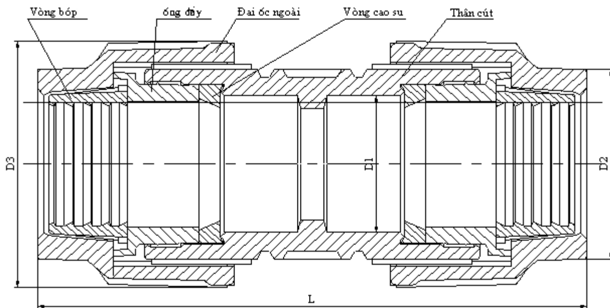
Hình 7: Bộ nối ống nhựa HDPEp kiểu giắc co
