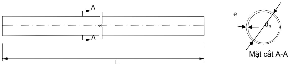
Hình 4 - Quy cách hình dáng ống nhựa HDPE p
