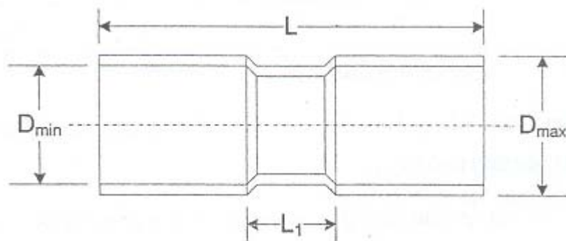
Hình 2 – Khớp nối thẳng có gờ
